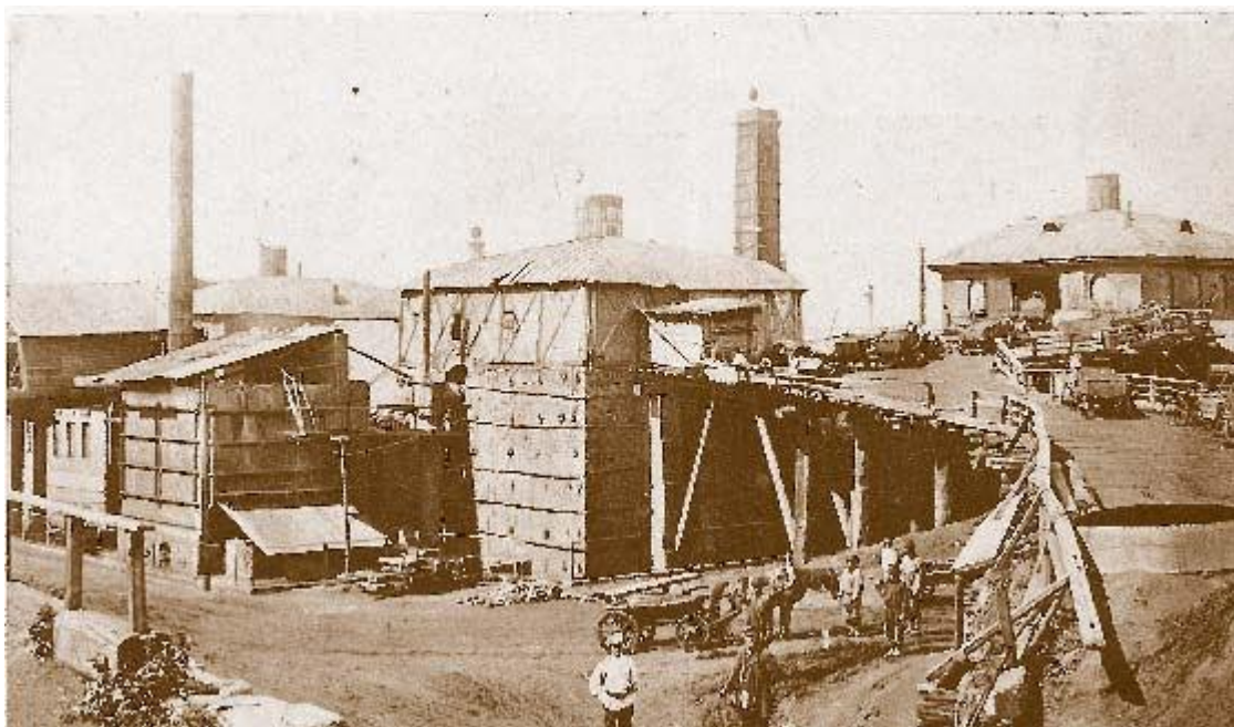
Одна из старинных доменных печей, бывших в Юрюзанском заводе
